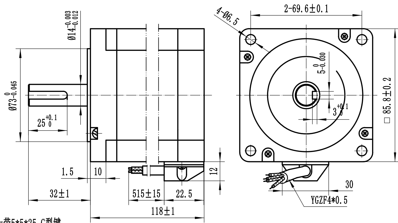
5*5*25C type key带5*5*25 C型键
